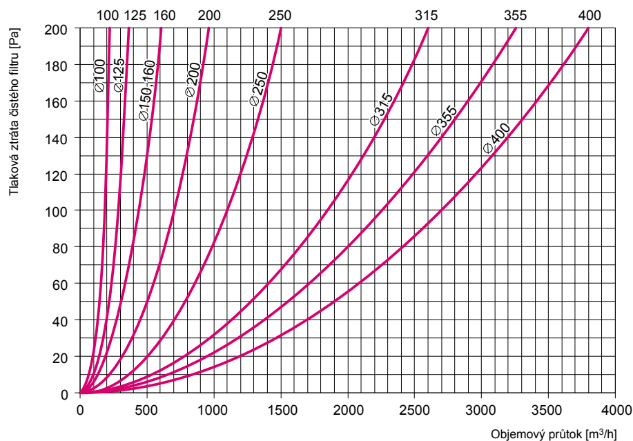
Graf tlakové ztráty filtračního boxu FLK-B s filtrační vložkou G4
