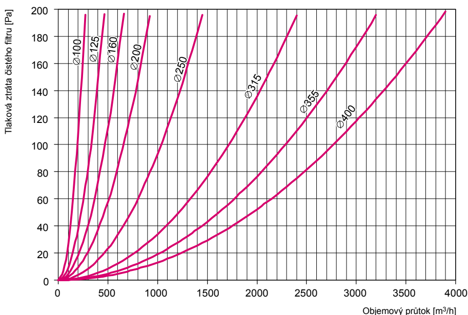
Graf tlakové ztráty filtračního boxu FLK-B s filtrační vložkou G3
