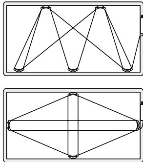
Příklad instalace kapiláry na straně vzduchu
